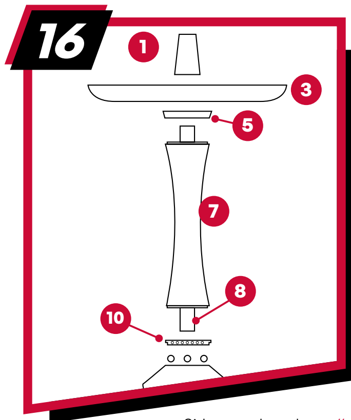
Sideways above base // Über der Base zur Seite
