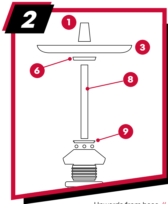
Upwards from base // Von Base nach oben
