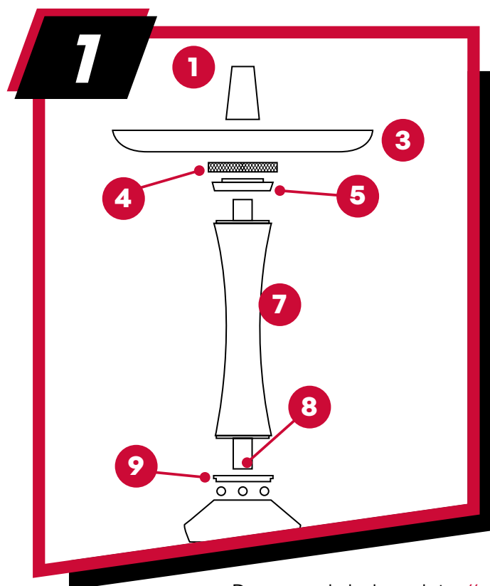
Downwards below plate // Unterm Teller nach unten
